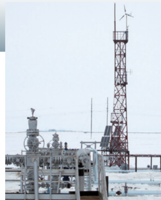
Рис. 1. Куст газовых скважин
